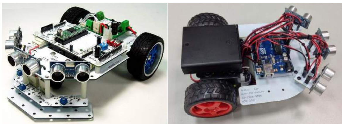
輪型機器人避障比賽參考作品
