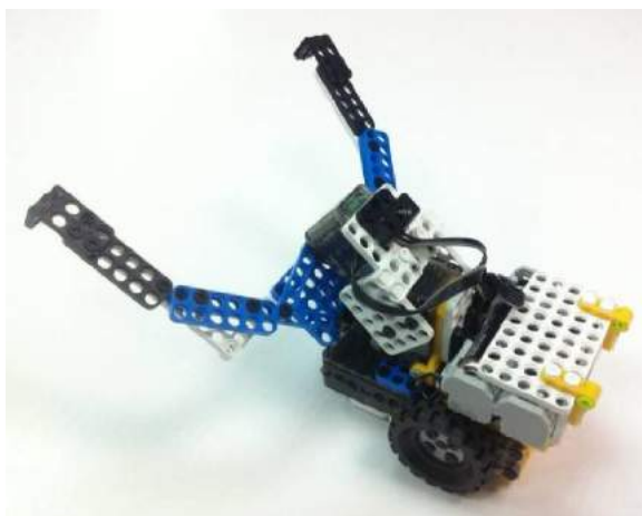
【圖三】自走車過三關比賽參考作品
